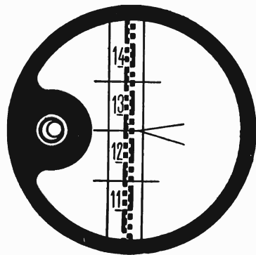
Рис. 36. Поле зрения нивелира NiB-5.
