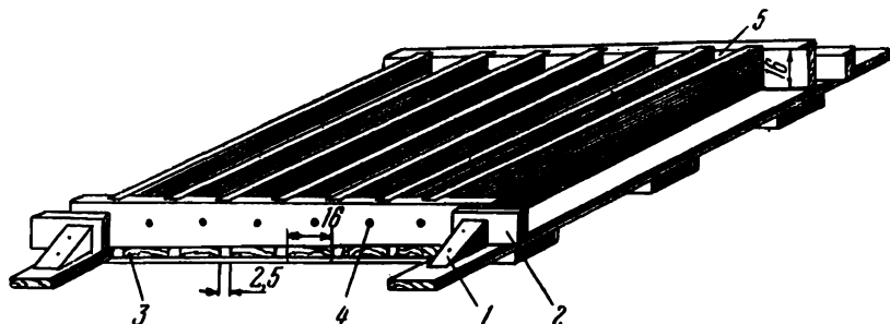
Рис. 21. Многаячейковая опалубка.
