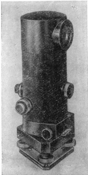
Рис. 32. Нивелир Ni007.
