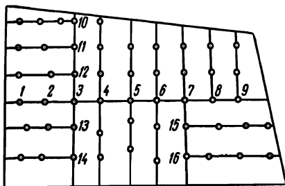
Рис. 72. Способ параллельных нитей.
