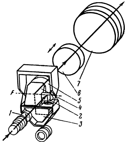
Рис. 37. Оптическая схема нивелира NiB. 1 — сетка нитей; 2, 3 и 4 — призмы компенсатора; 5, 6 и 7 — линзы объектива.
