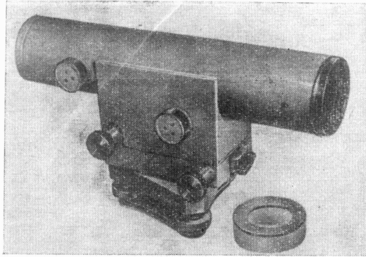
Рис. 27. Нивелир Н2.
