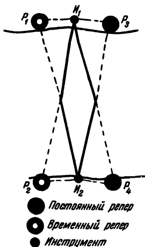
Рис. 69. Передача через препятствия шириной более 200 м.
