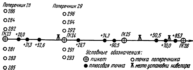
Рис. 71. Участок линии технического нивелирования.
