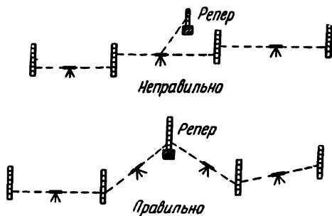
Рис. 63. Привязка к нивелирным знакам.
