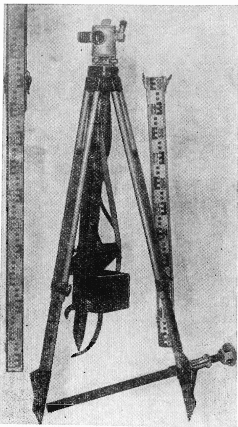
Рис. 44. Комплект нивелира ТН-6.
