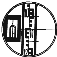
Рис. 22. Нивелир НЗ.
