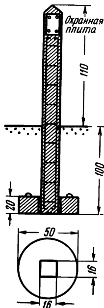
Рис. 12. Железобетонный опознавательный столб.
