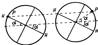
Рис. 56. Проверка горизонтальной нити нивелира.
