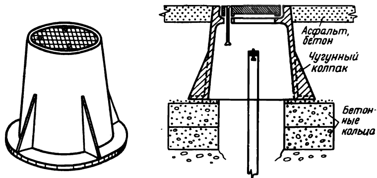
Рис. 15. Чугунный колпак (ковер).
