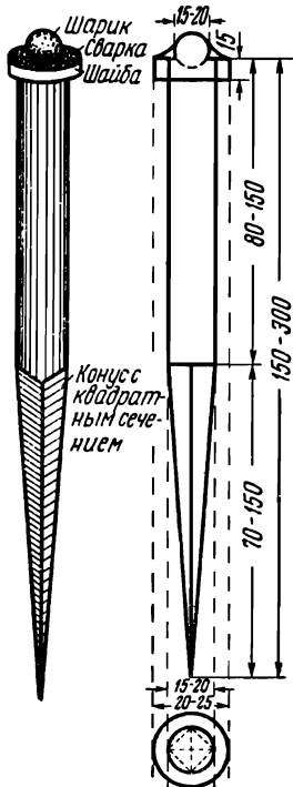
Рис. 52. Металлический костыль.
