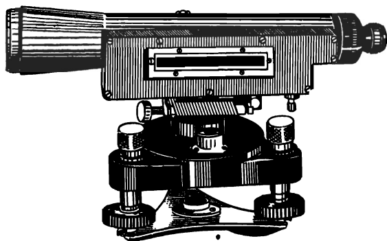
Рис. 26. Нивелир НГ.
