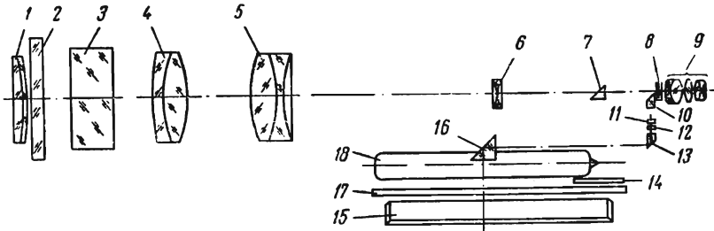
Рис. 28. Оптическая схема нивелира Н2.
