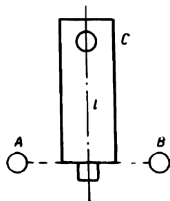
Рис. 54. Определение цены деления круглого уровня.
