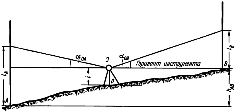
Рис. 85. Измерение превышений тригонометрическим нивелированием методом из середины.
