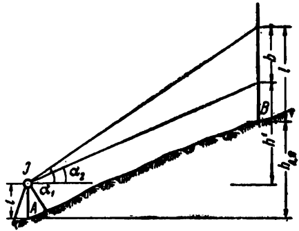
Рис. 86. Измерение превышения методом на две высоты.
