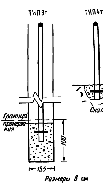
Рис. 17. Реперы для закрепления линий технического нивелирования, закладываемые бурением (3т) и в скальную породу (4т).
