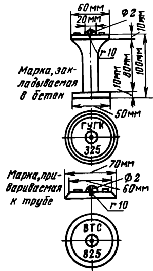
Рис. 10. Марки для грунтовых реперов.
