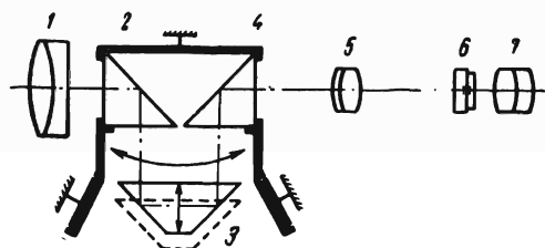
Рис. 46. Оптическая схема нивелира Ni050. 1 и 5 — линзы объектива; 2, 3 и 4 — призмы компенсатора; 6 — сетка нитей; 7 — окуляр.
