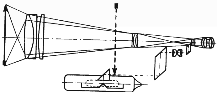
Рис. 43. Оптическая схема нивелира НТ.
