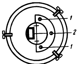
Рис. 55. Крепление сетки нитей нивелира НВ-1.
