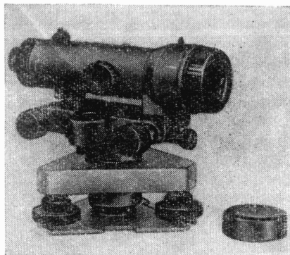
Рис. 23. Нивелир НВ-1.
