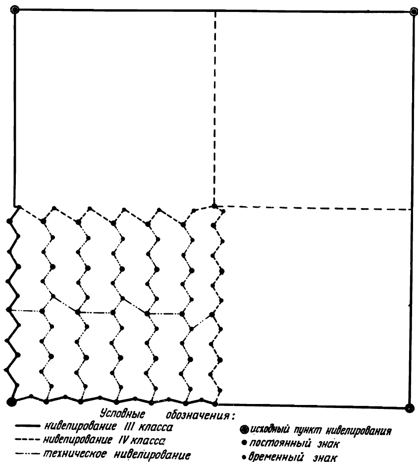
Рис. 4. Схема нивелирной сети на объекте площадью около 1000 км 2 .
