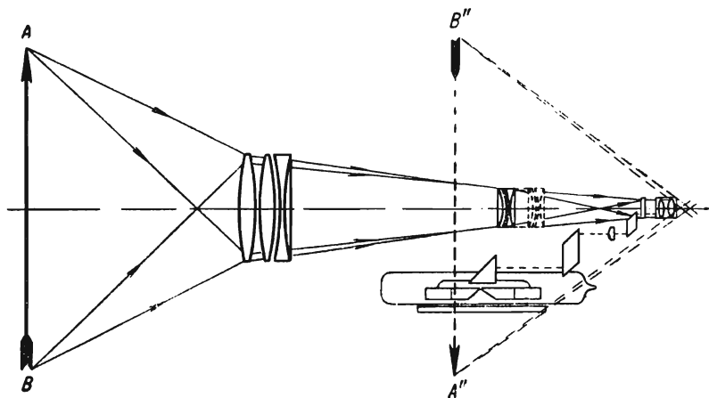
Рис. 25. Оптическая схема нивелира НЗ.
