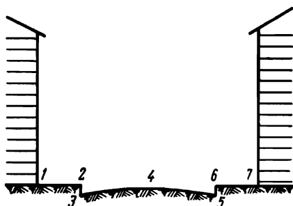
Рис. 80. Места установок реек при нивелировании улицы.
