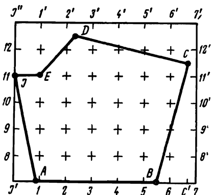
Рис. 75. Разбивка квадратов.
