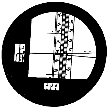
Рис. 30. Поле зрения нивелира Н2.
