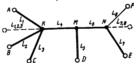
Рис. 93. Уравнивание сети нивелирных линий методом эквивалентной замены.
