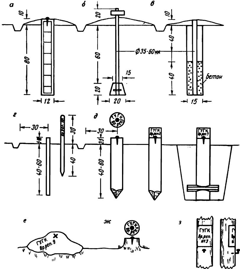
Рис. 20. Временные реперы для зоны сезонного промерзания:
