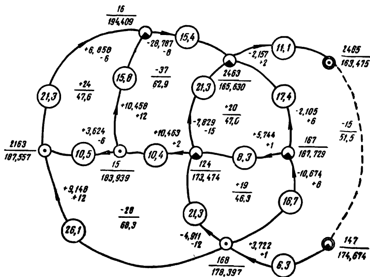
Рис. 89. Уравнивание нивелирной сети методом полигонов.
