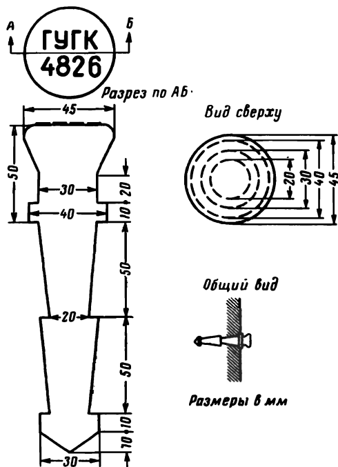
Рис. 7. Стенной репер.
