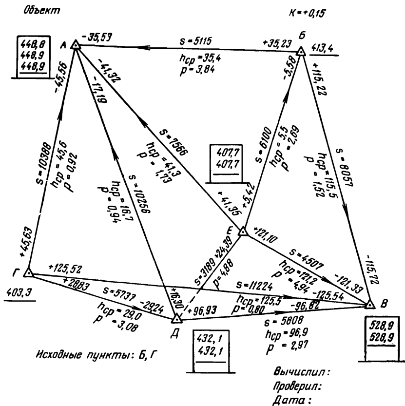
Рис. 92. Схема уравнивания высот пунктов триангуляции.
