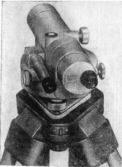
Рис. 35. Нивелир NiB-5.
