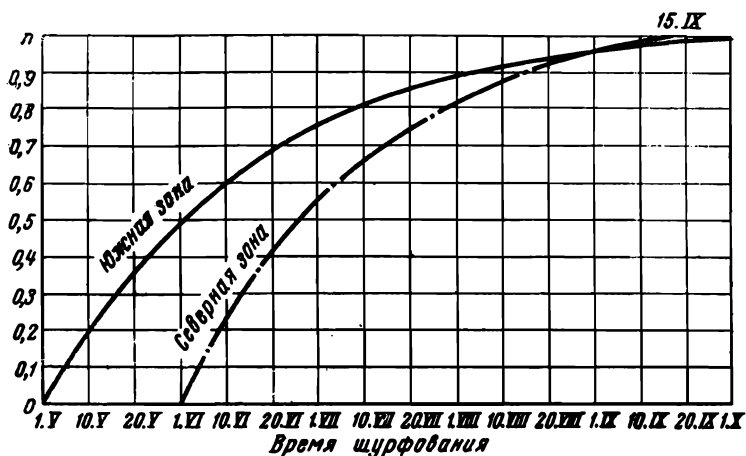
Рис. 6. График для определения показателя протаивания.
