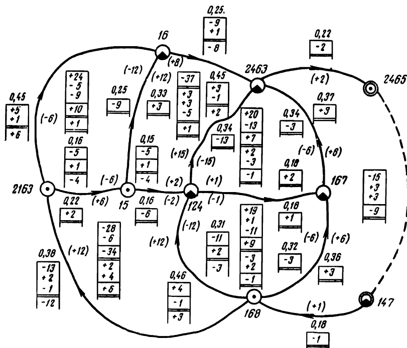
Рис. 90. Уравнивание нивелирной сети методом полигонов.
