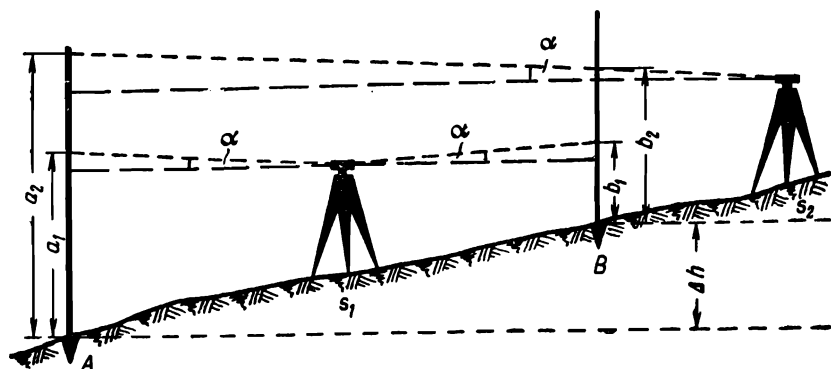
Рис. 58. Определение угла i нивелира вторым способом.
