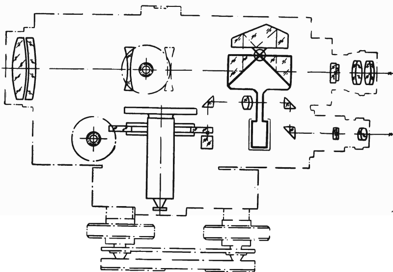
Рис. 41. Оптическая схема нивелира Ni025.
