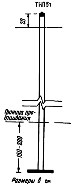
Рис. 18. Репер для закрепления линий технического нивелирования, закладываемый бурением в зоне многолетней мерзлоты.
