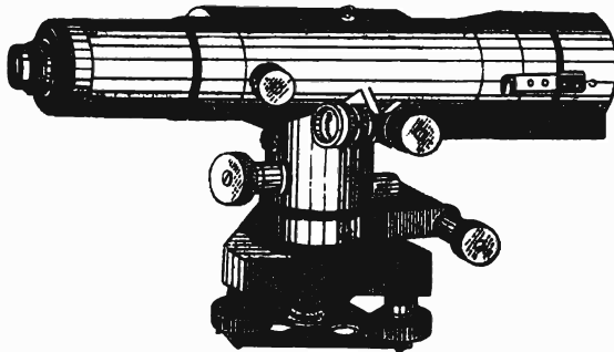
Рис. 29. Нивелир НА-1.
