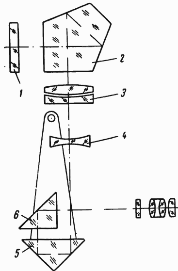
Рис. 33. Оптическая схема нивелира Ni007
