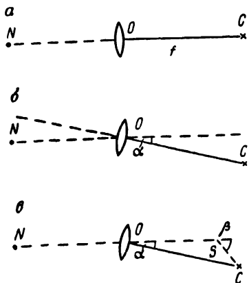
Рис. 31. Принцип работы нивелира с компенсатором.
