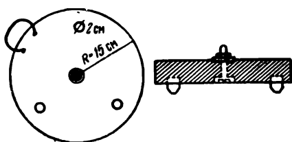
Рис. 53. Деревянный башмак.
