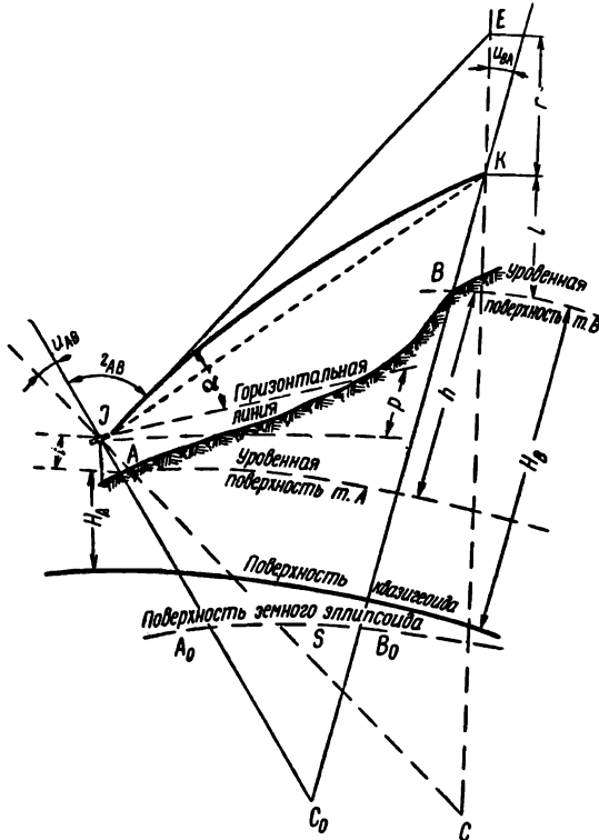
Рис. 83. Определение превышения методом тригонометрического нивелирования.
