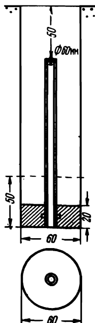
Рис. 13. Грунтовый репер нивелирной сети I—IV классов для северных труднодоступных районов зоны сезонного промерзания грунтов.
