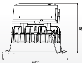
Габаритные размеры (мм)
