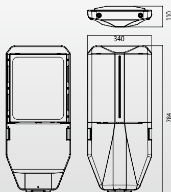
Габаритные размеры (мм)
