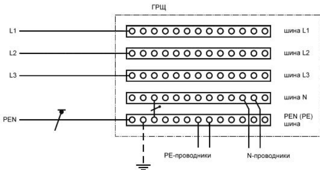
Рисунок 54.1a - Пример 1
