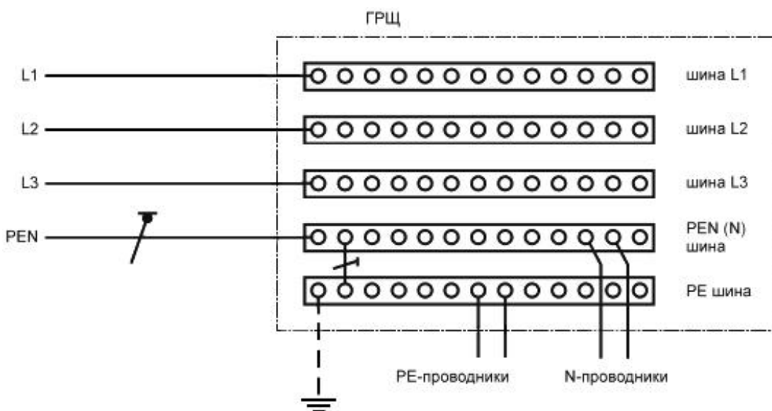
Рисунок 54.1b - Пример 2
