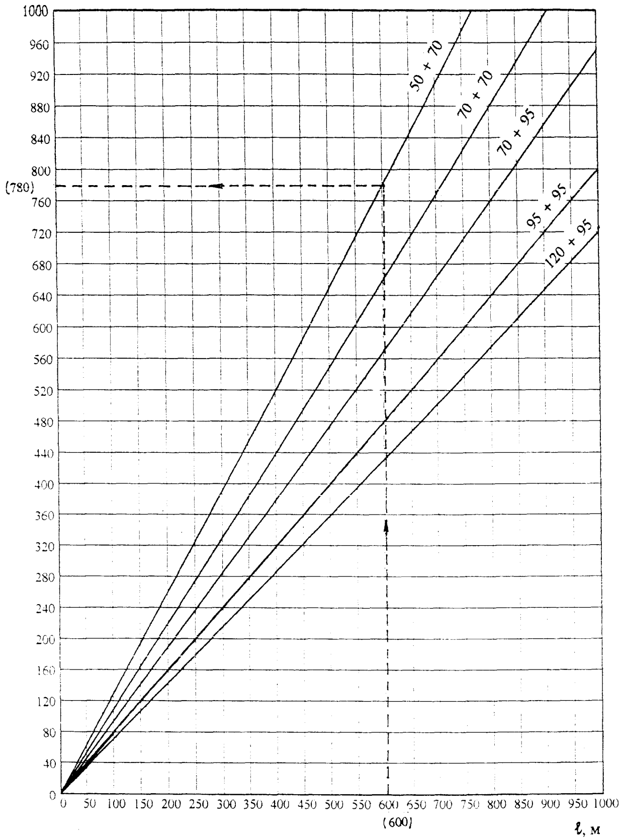
2. График определения Z_{\text{ит}} СИП ( \phi+0 ) сечением 50+70; 70+70; 70+95; 95+95; 120+95, марок 1, 1А, 2 и 2А.
