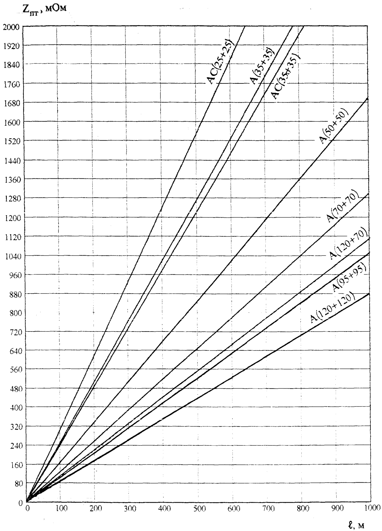
3. График определения Z_{\text{пт}} неизолированных (голых) проводов ( \phi+0 )
