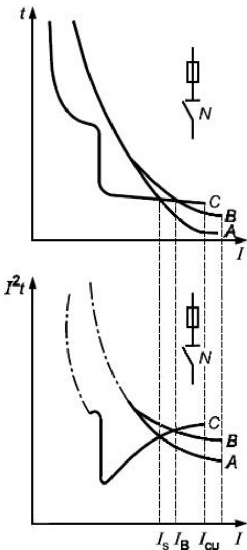
Рисунок D.1 - Координация по сверхтокам между автоматическим выключателем и предохранителем или резервной защитой, осуществляемой предохранителем. Рабочие характеристики
