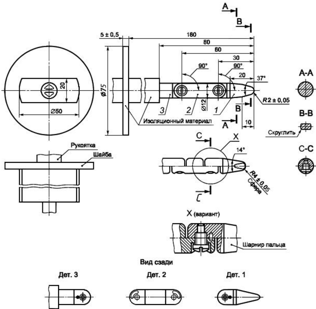
Рисунок 9 - Стандартный испытательный палец
