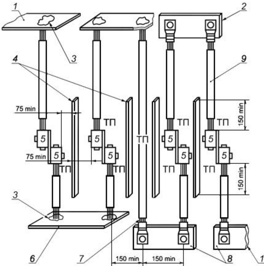
Рисунок L.1 - Испытательное устройство
