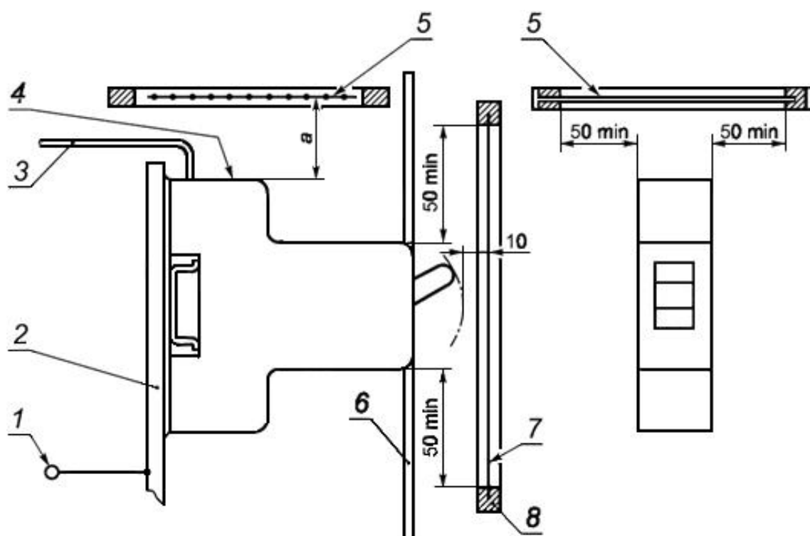
Рисунок Н.1 - Испытательное устройство
