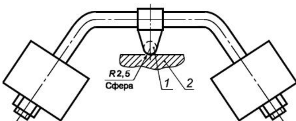
Рисунок 16 - Установка для испытаний давлением шарика
