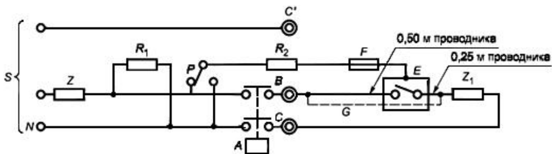
Рисунок 3 - Однополюсный автоматический выключатель
