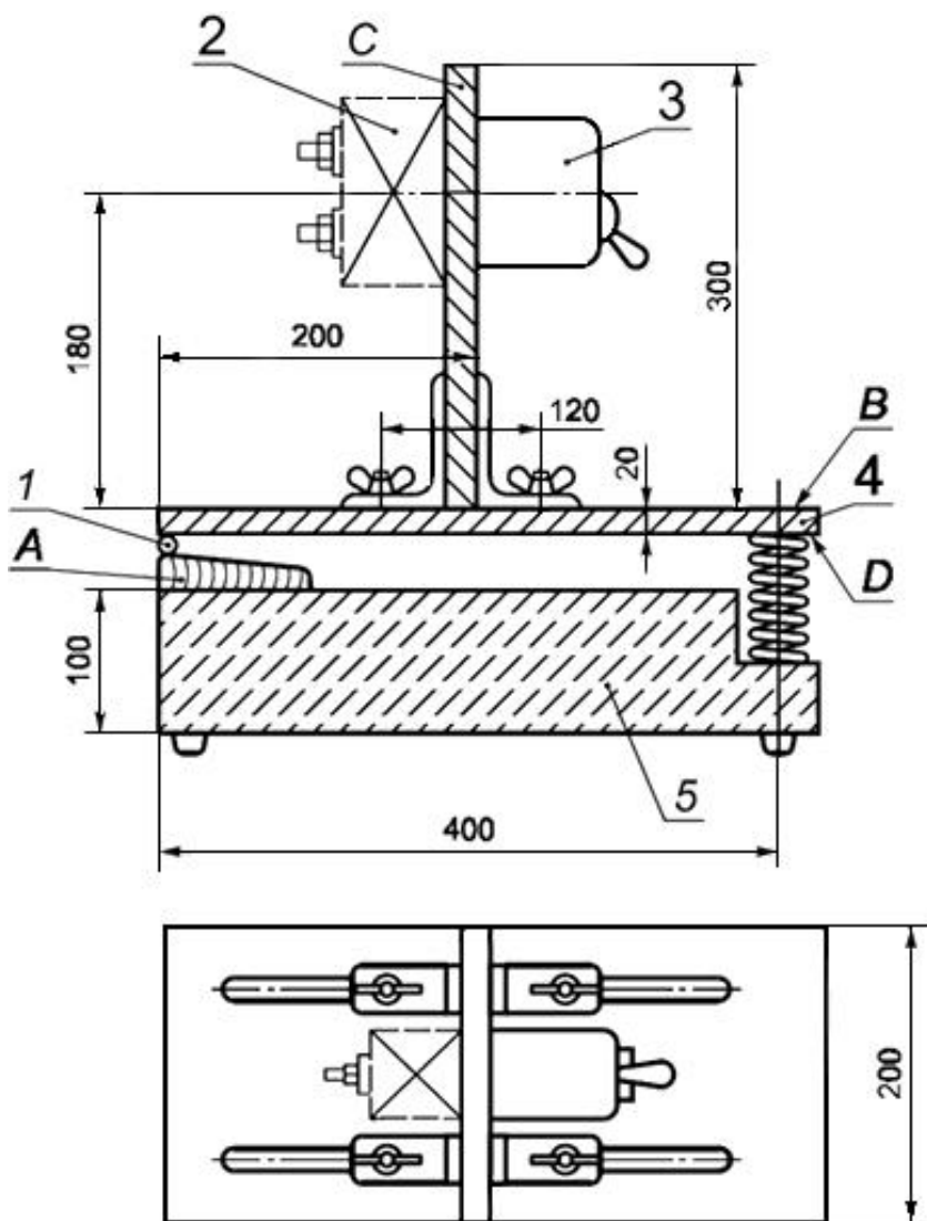
Рисунок 8 - Устройство для испытаний на механический толчок
