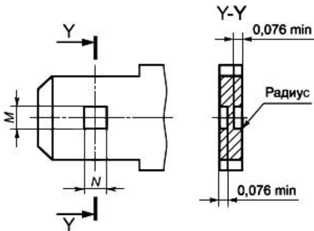
Рисунок К.4 - Размеры прямоугольных размеров фиксации
