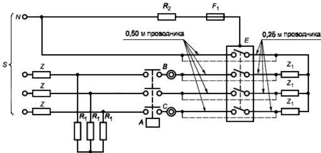
Рисунок 6 - Четырехполюсный автоматический выключатель
