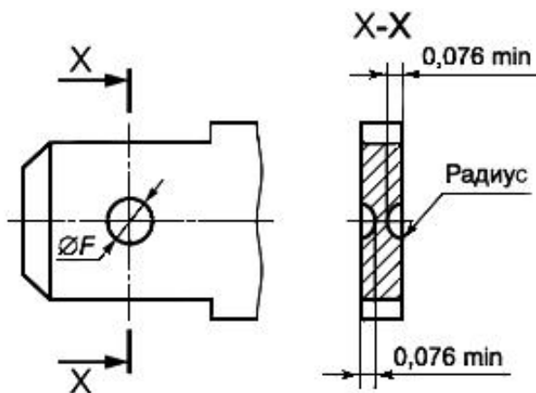
Рисунок К.3 - Размеры круглых углублений фиксации
