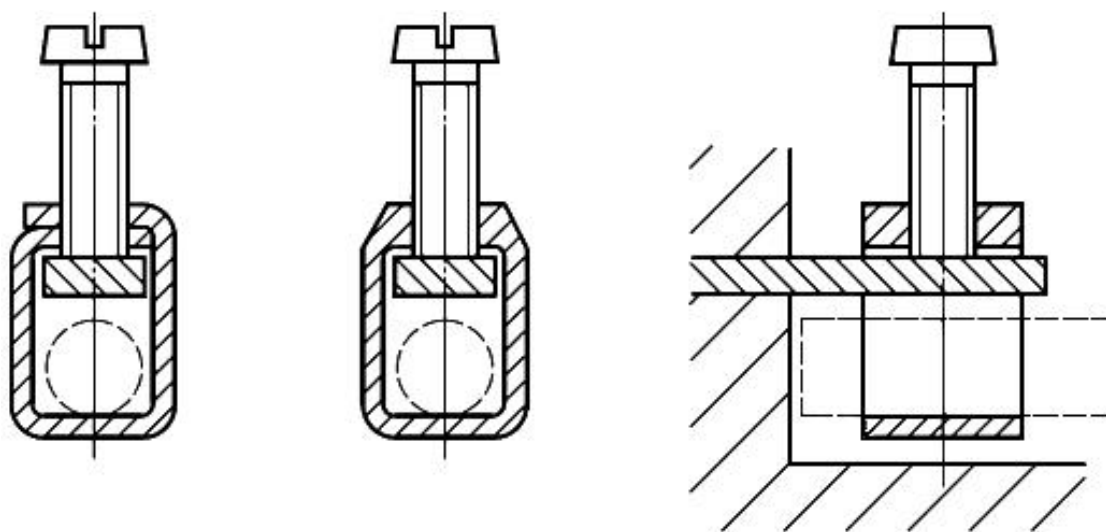
Рисунок F.1 - Примеры столбчатых выводов
