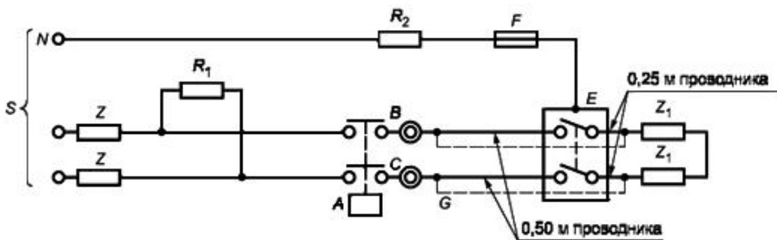
Рисунок 4б - Двухполюсный автоматический выключатель с двумя защищенными полюсами
