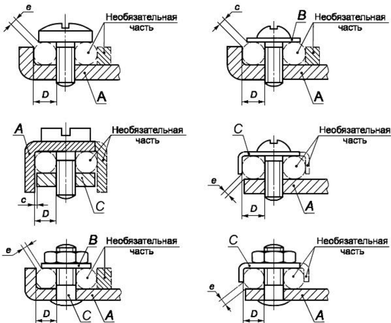
Рисунок F.2 - Пример винтовых и штыревых выводов
