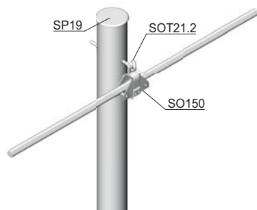
Анкерная опора
