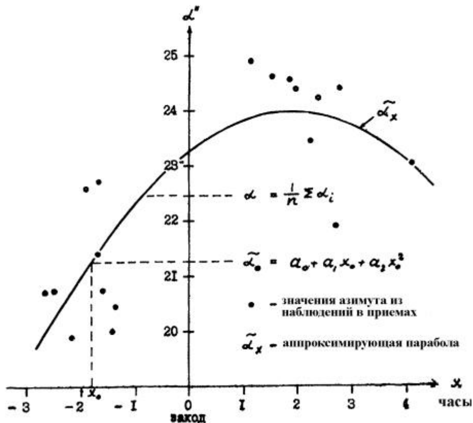
Рис. 1. Изменение значений азимута в приемах под воздействием суточного хода боковой рефракции
