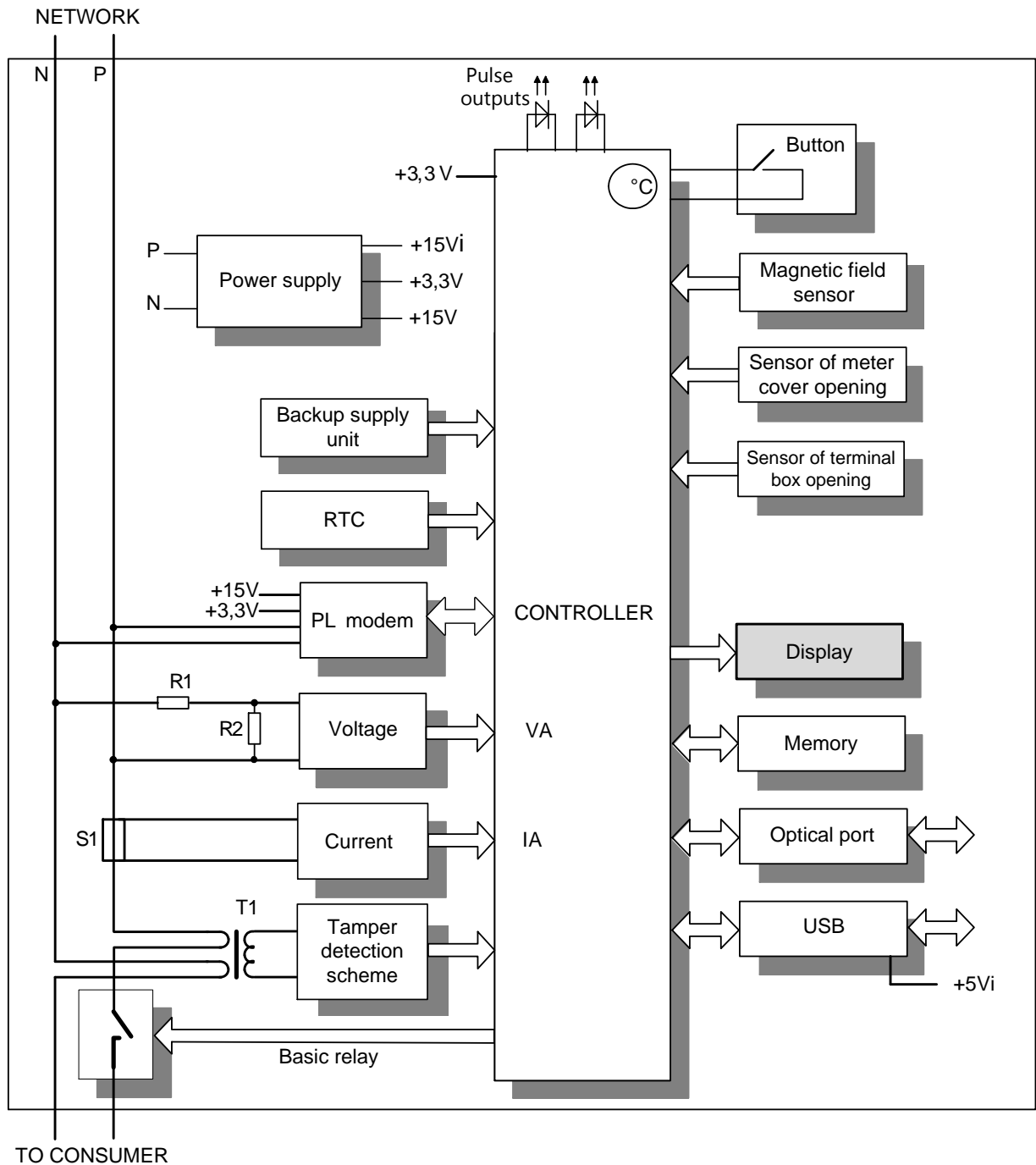
б) Однофазный счетчик
