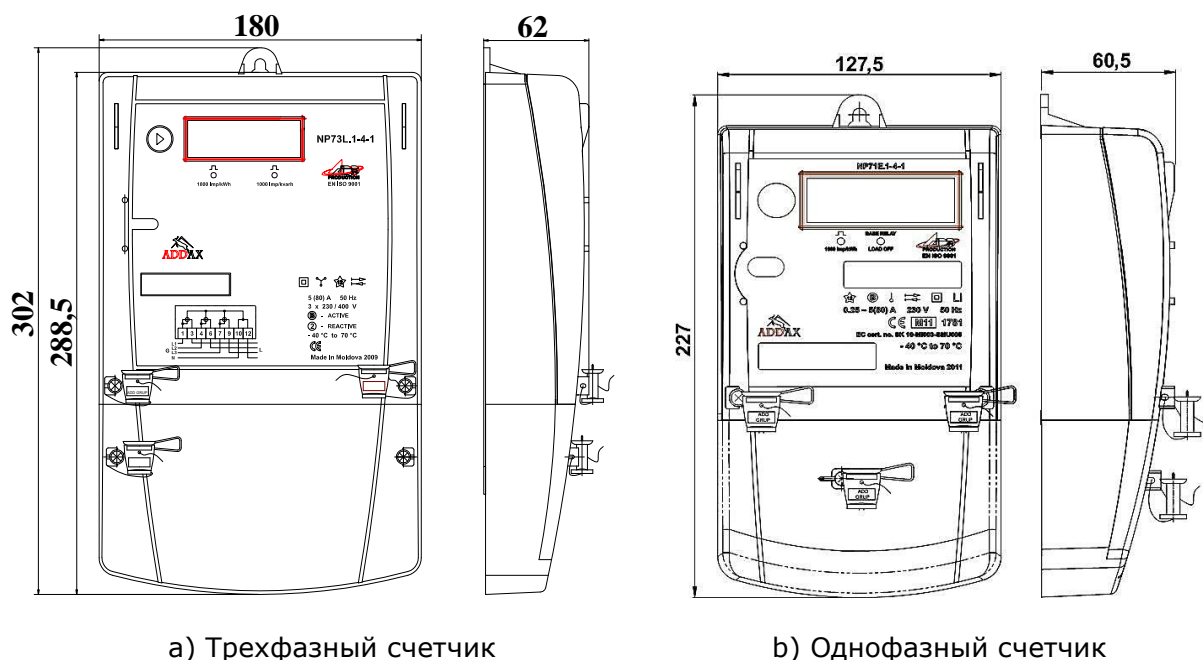
Рис. 4.4. Общий вид и габаритные размеры счетчика со стандартной крышкой клеммника
