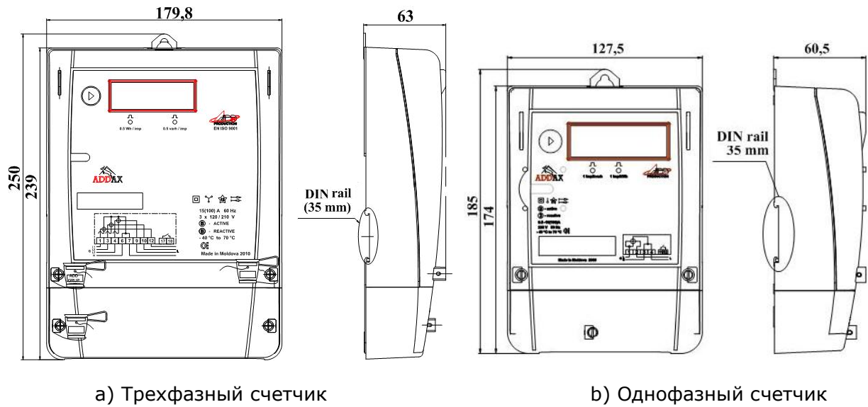
Рис. 4.5. Общий вид и габаритные размеры счетчика с укороченной крышкой клеммника
