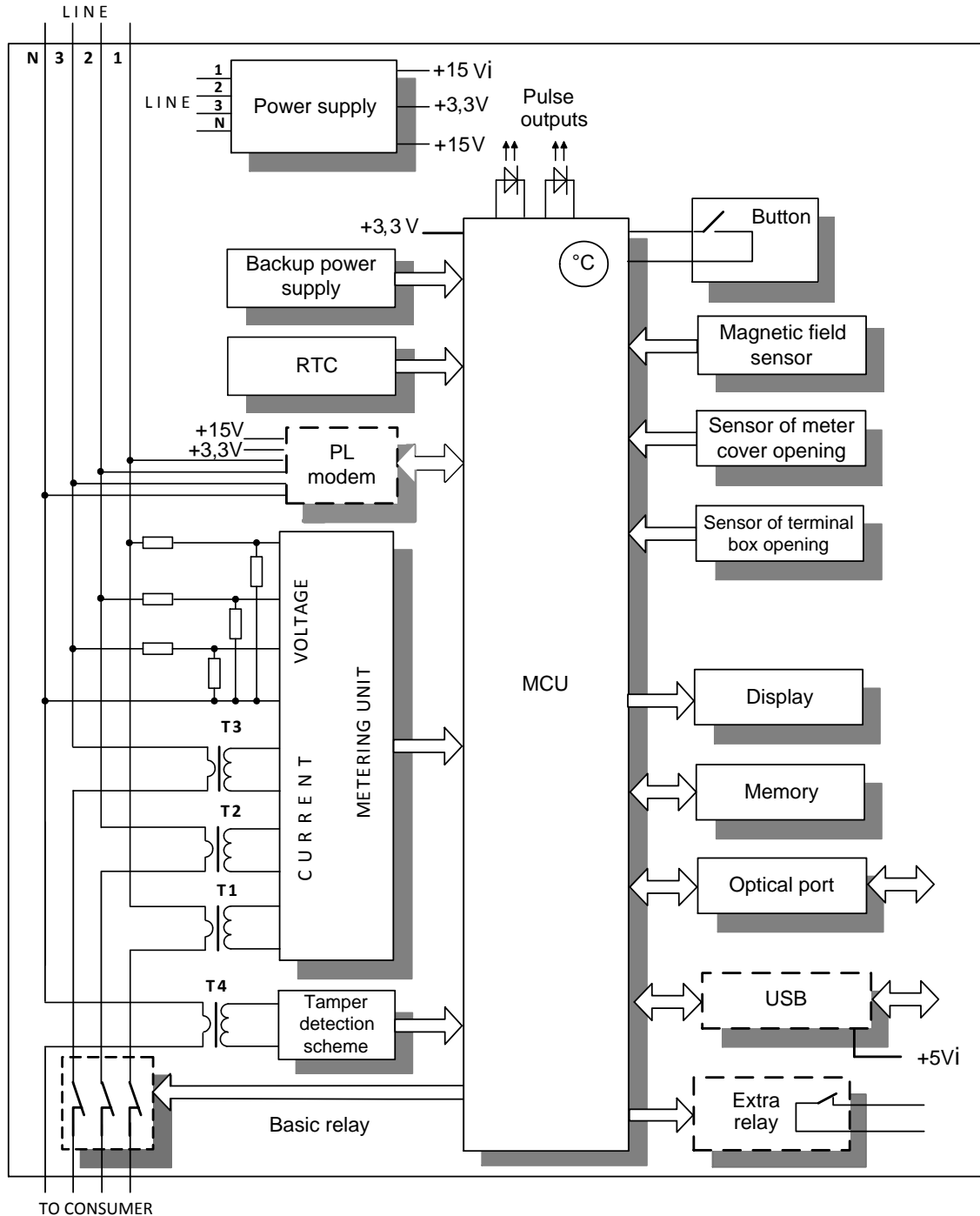
а) Трехфазный счетчик
