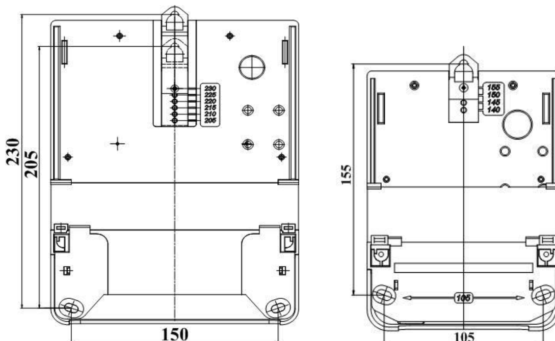
а) Трехфазный счетчик
