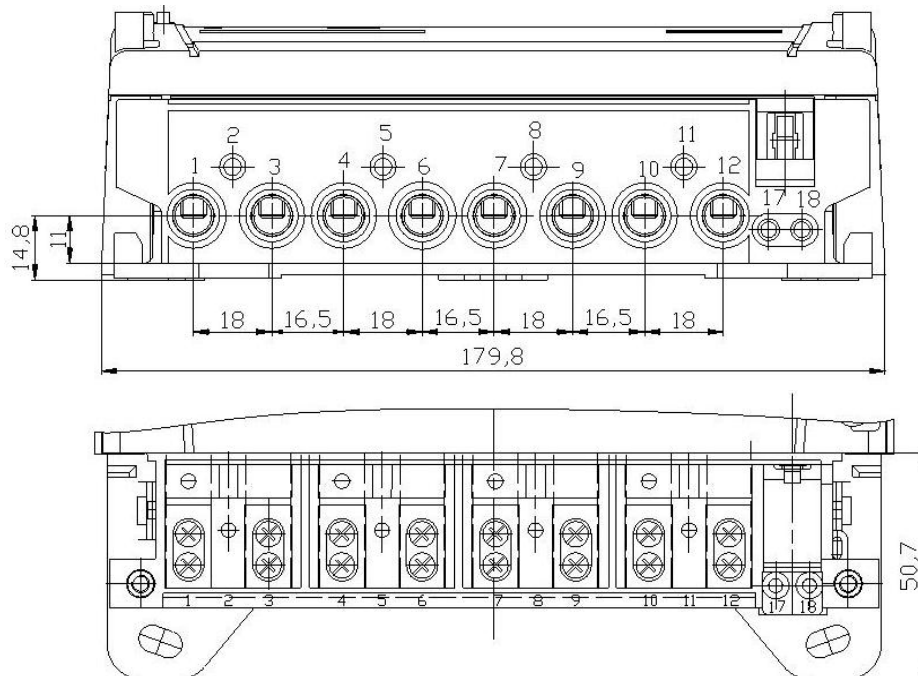
Рисунок 4.6. Клеммник трехфазного счетчика
