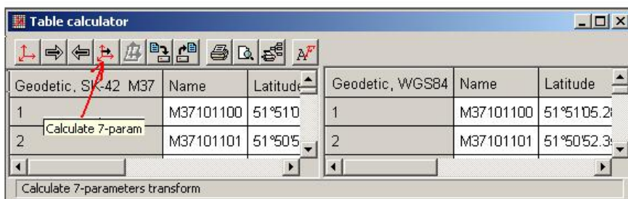
Рис. П5.9 Вид окна с преобразованными координатами WG 84 правой панели
