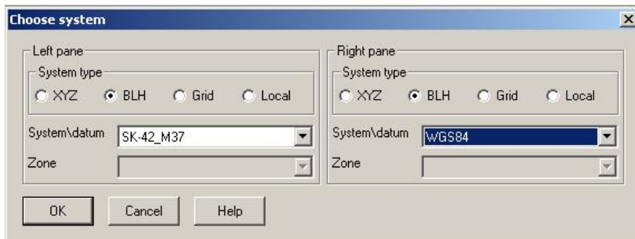
Рис. П5.8 Вид окна после выбора для правой панели системы координат WGS 84
