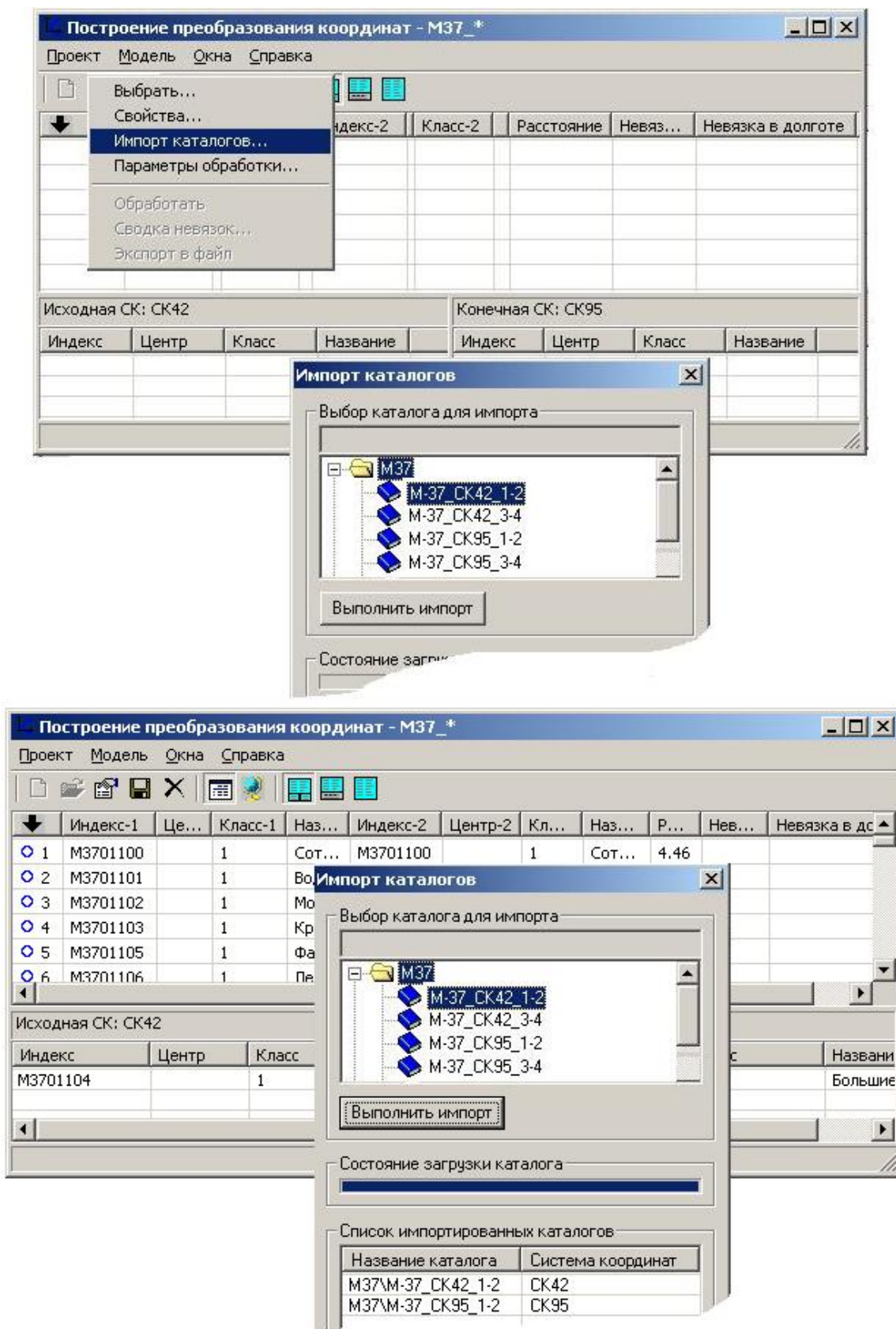
Рис. ПЗ.9 Вид окон при импорте координат из каталогов в проект из каждой из систем координат
