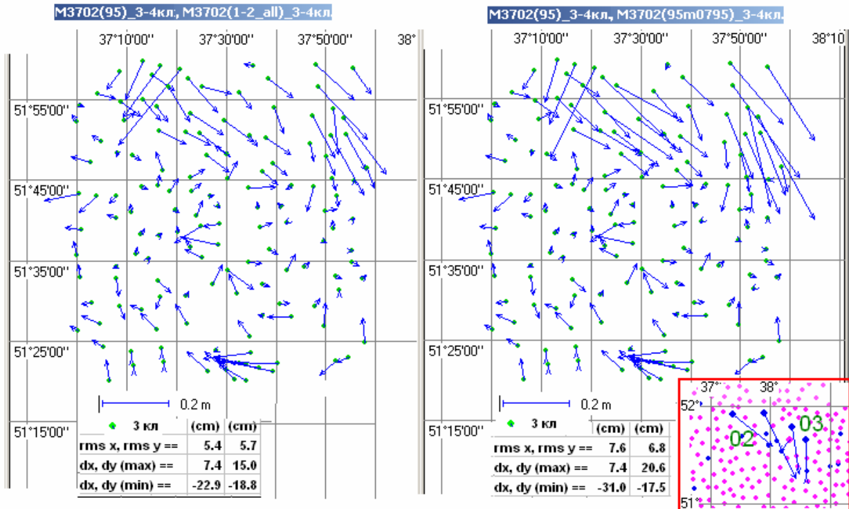
Рис. П4.5 а Трапеция М3702 (м-б 1:200000)
