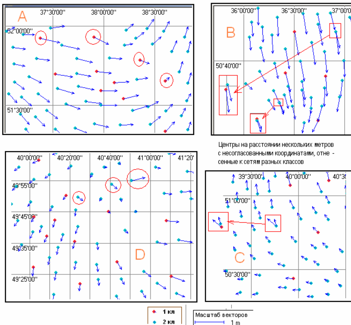
Рис. Пб.2А,В,С,Д. Деформации ГГС в СК42 на отдельных участках листа М37.
