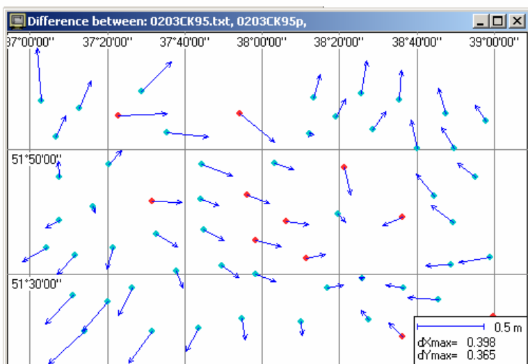
Рис.Пб.3б. Остаточные расхождения координат на тр. М3702 и М3703
