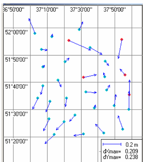
Рис. Пб.4. Остаточные уклонения координат. Трапеция М3702
