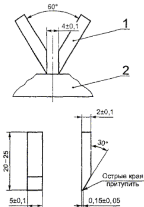
1 - электрод; 2 - образец
