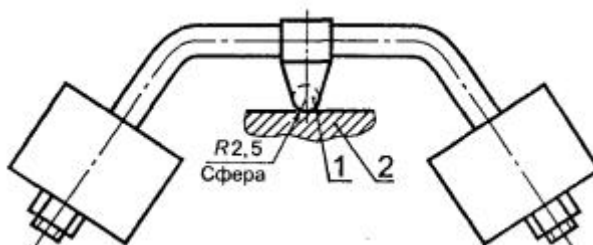
Рисунок 12 - Установка для испытания на сжатие
