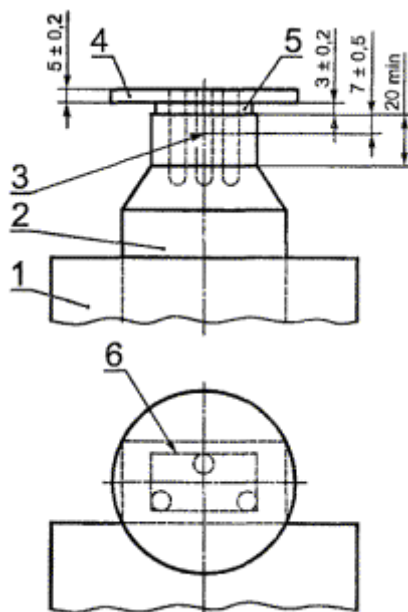
Рисунок 13 - Установка для испытания на истирание изоляционных трубок штырями вилок
