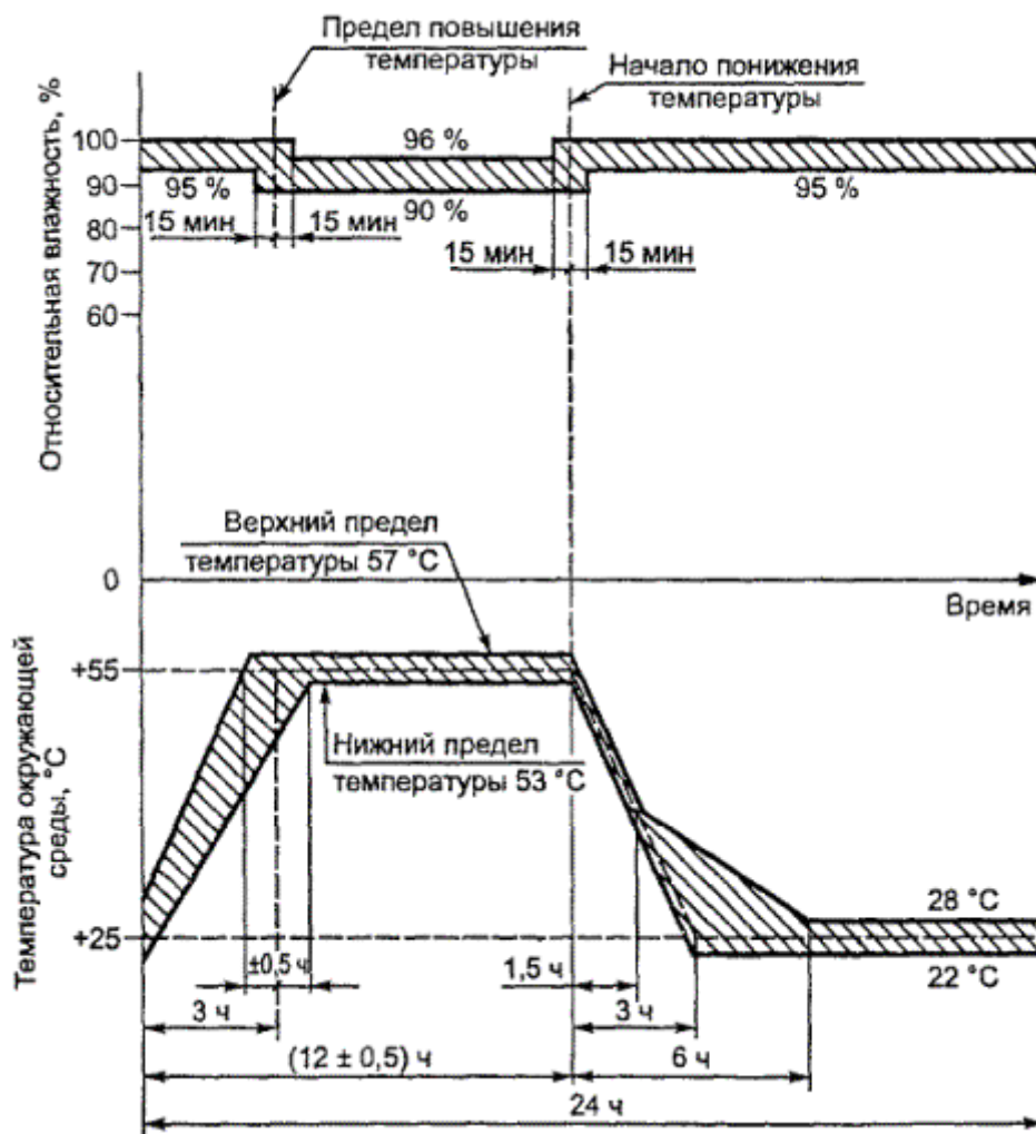
Рисунок 22 - Цикл испытания на надежность (9.22.1.3)
