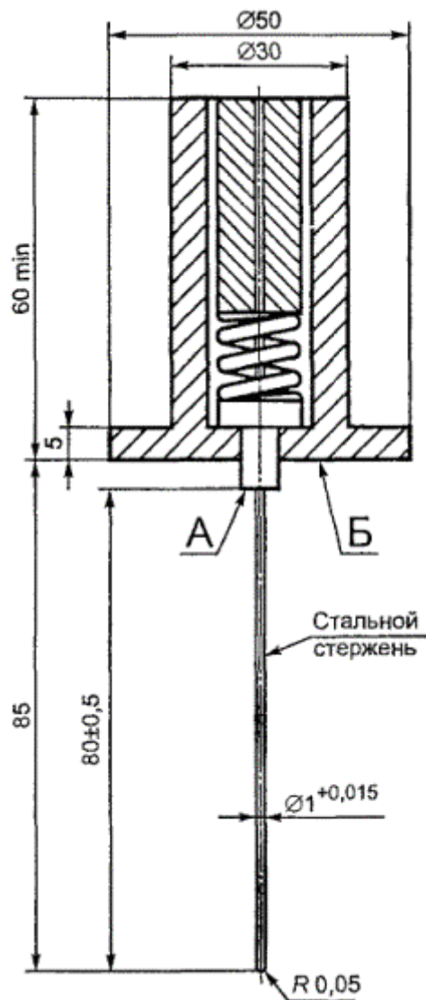
Рисунок 3 - Измерительный прибор для проверки недоступности токоведущих частей
