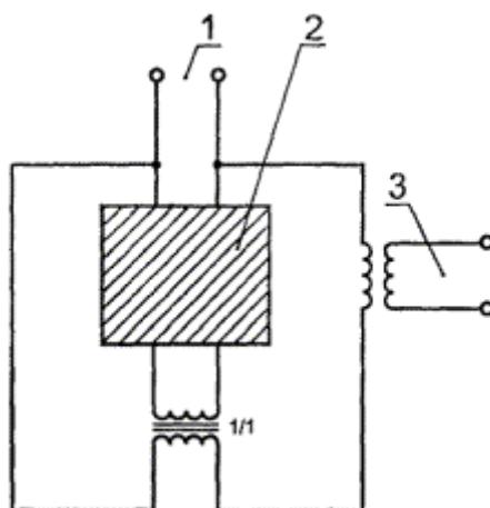
1 - источник питания при напряжении, равном 1,1U_n ; 2 - испытуемое УЗО-ДП; 3 - источник тока
