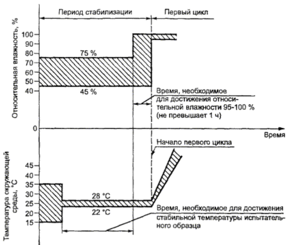
Рисунок 21 - Период стабилизации при испытании на надежность (см. 9.22.1.3)
