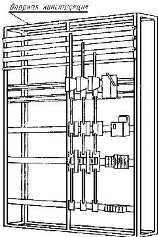
НКУ заводского изготовления открытого типа
