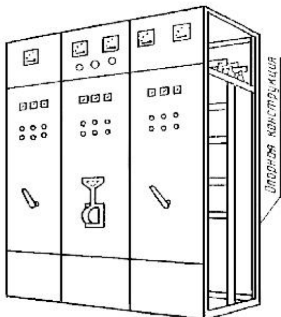
НКУ заводского изготовления открытого типа, защищенное спереди
