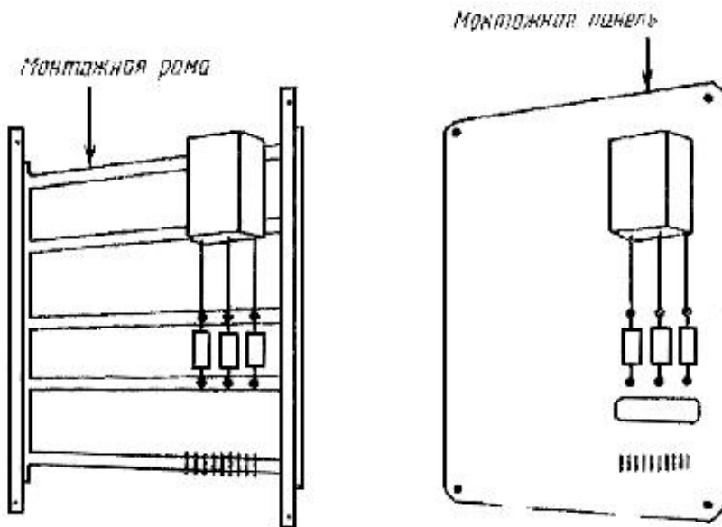
Неподвижные части
