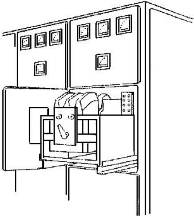
Выдвижная часть
