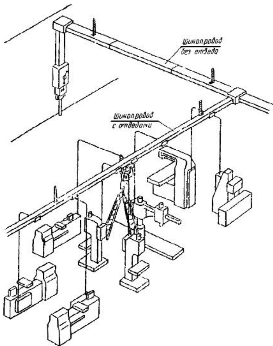
Система сборных шин (шинопровод)
