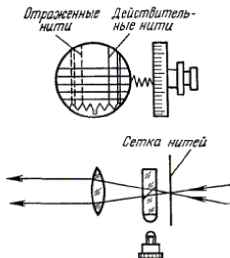
Рис. 10.50. Поле зрения микрометра и ход лучей в автоколлимационном окуляре
