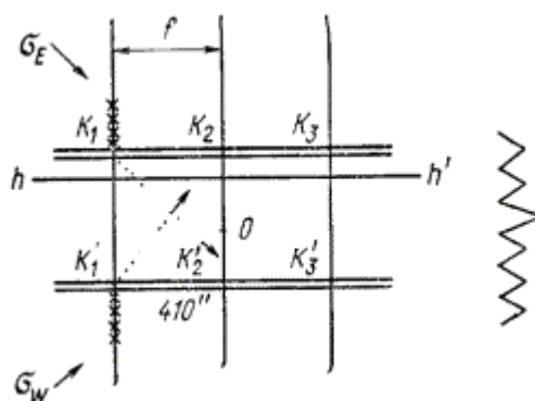
Рис. 3.4. Сетка нитей контактного микрометра теодолита АУ 2/10
