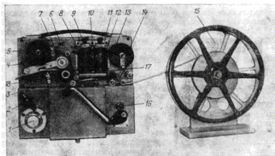
Рис. 10.29. Маркопечатающий хронограф ХПМ-3
