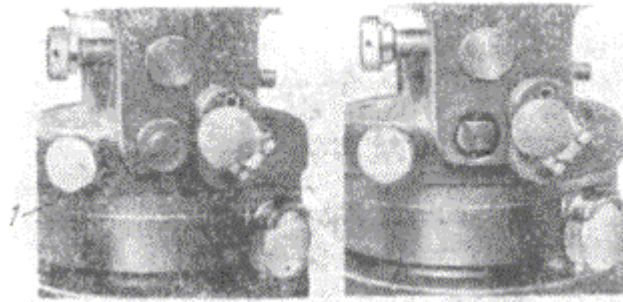
Рис. 11.1. Доступ к юстировочным винтам уровня при алидаде горизонтального круга теодолита ДКМЗ-А
