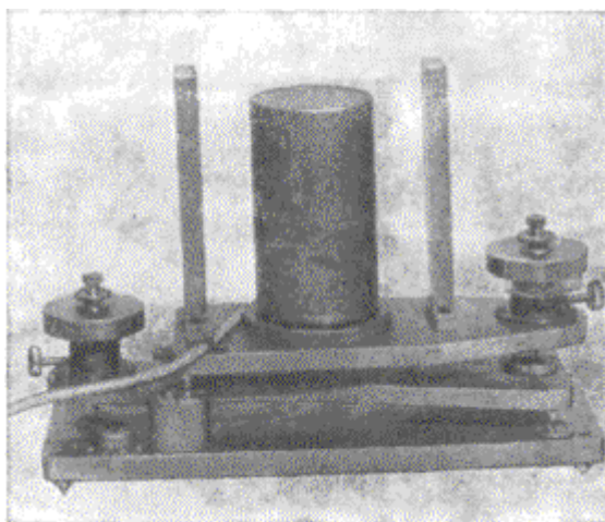
Рис. 10.45. Полевой экзаменатор
