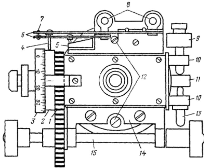
Рис. 10.3. Схема контактного микрометра астрономического универсального теодолита АУ 2/10:
