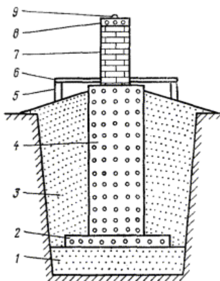
Рис. 2.1. Астрономический столб
