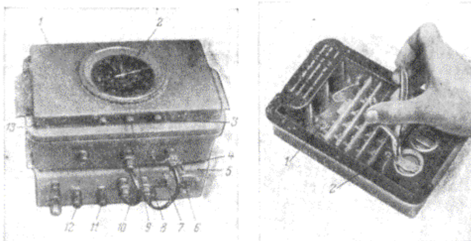
Рис. 10.26. Кварцевый хронометр «Chronotome CP»
