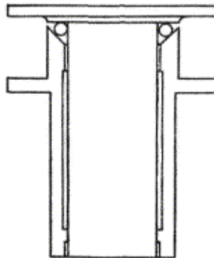
Рис. 10.13. Кинематическая схема вертикальной оси теодолита Т4
