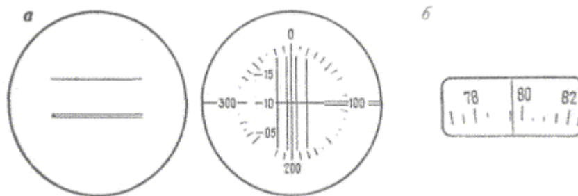
Рис. 10.19. Поле зрения контактного микрометра:
