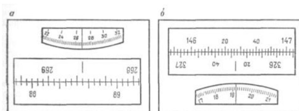
Рис. 10.11. Поле зрения оптических микрометров:
