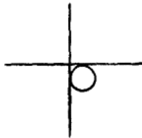
Рис. 9.2. Положение Солнца в момент наблюдения
