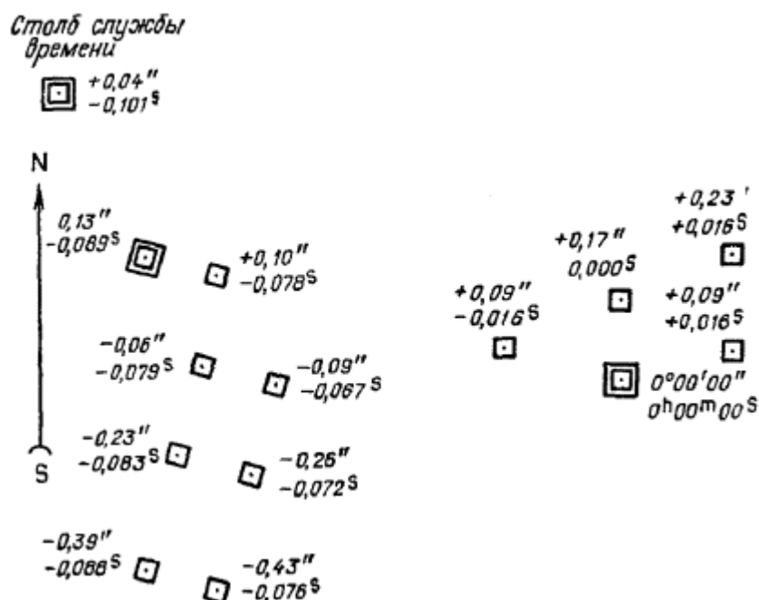
Рис. 3.3. Схема расположения столбов (Ташкент)
