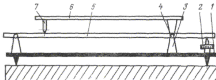
Рис. 10.42. Кинематическая схема составного экзаменатора
