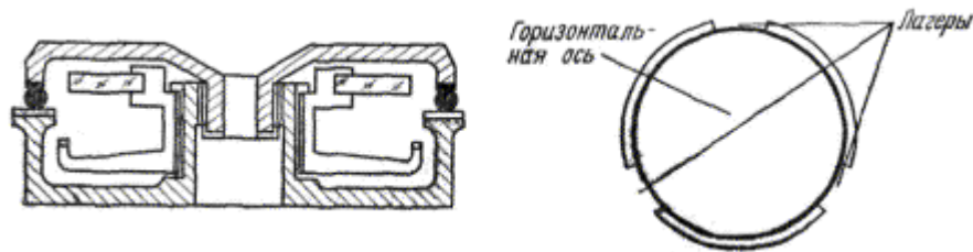
Рис. 10.21. Кинематическая схема вертикальной оси теодолита ДКМЗ-А
