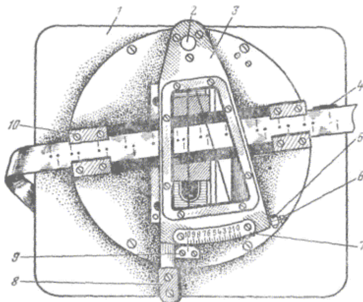
Рис. 10.33. Прибор для расшифровки хронограмм
