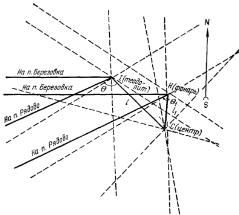
Рис. 8.1. Центрировочный лист
