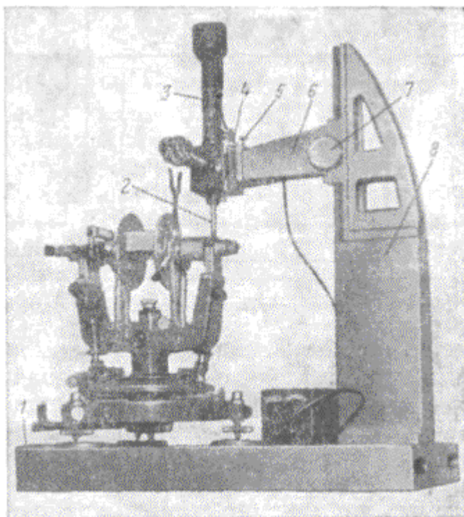
Рис. 10.40. Прибор для исследования цапф контактным способом
