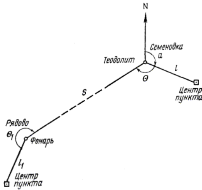
Рис. 8.2. Схема определения элементов центрировки и редуции
