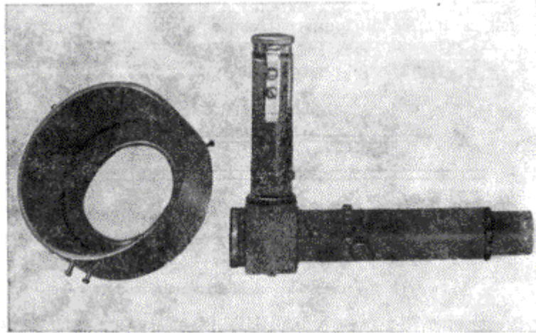
Рис. 10.41. Автоколлимационное устройство для исследования бокового гнутия
