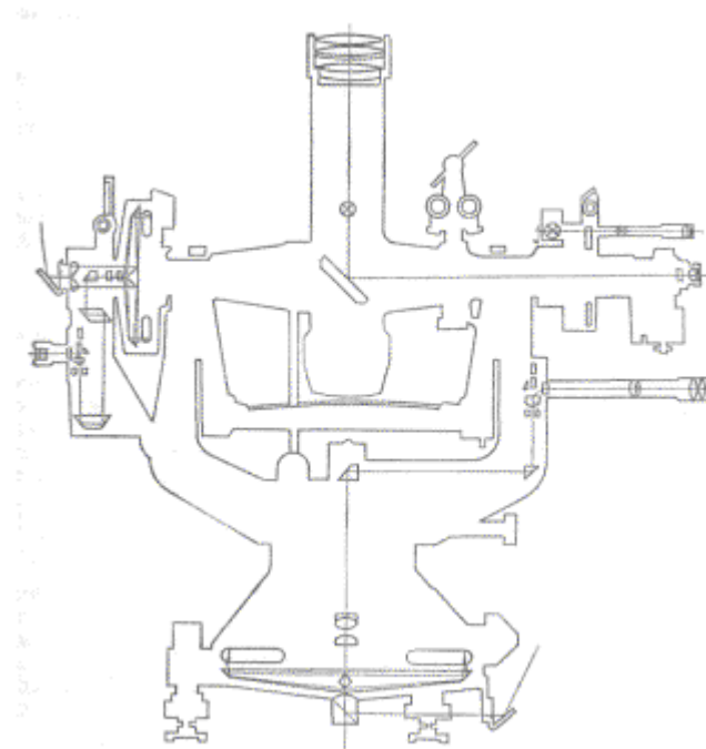
Рис. 10.10. Оптическая схема теодолита Т4
