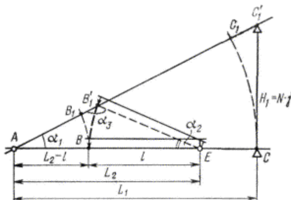
Рис. 10.43. Геометрическая схема составного экзаменатора
