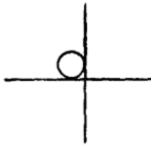
Рис. 9.1. Положение Солнца в момент наблюдения
