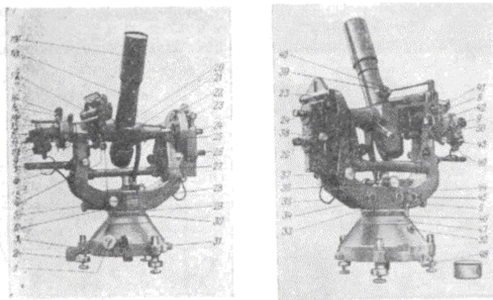
Рис. 10.6. Теодолит Вильд Т4. Вид со стороны наводящего винта горизонтального круга:
