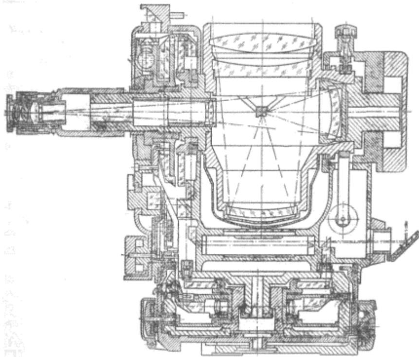
Рис. 10.18. Оптико-механическая схема теодолита ДКМЗ-А
