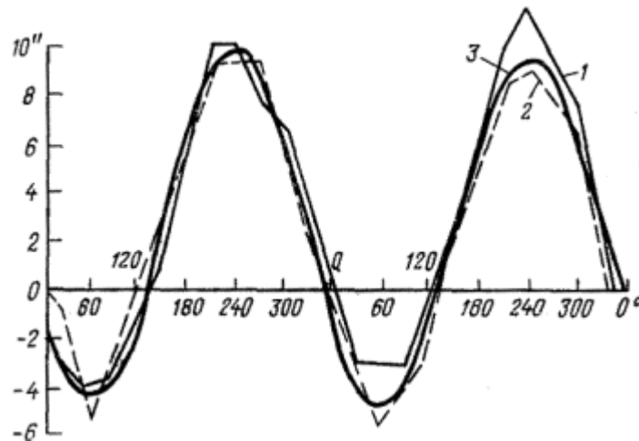
Рис. 11.4. График эксцентриситета алидады горизонтального круга:
