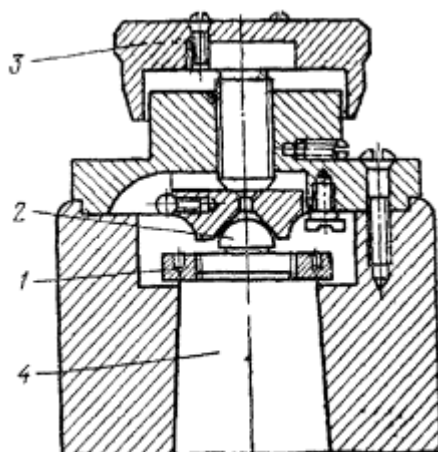
Рис. 10.5. Регулировочный конец вертикальной оси АУ 2/10:
