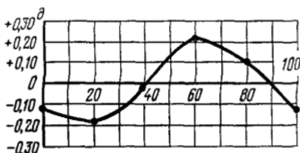
Рис. 11.6. График поправок за периодические погрешности винта микрометра
