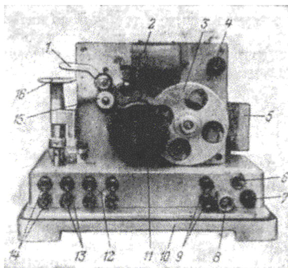
Рис. 10.31. Ленточный царапающий хронограф типа М 427 фирмы «Favag»:
