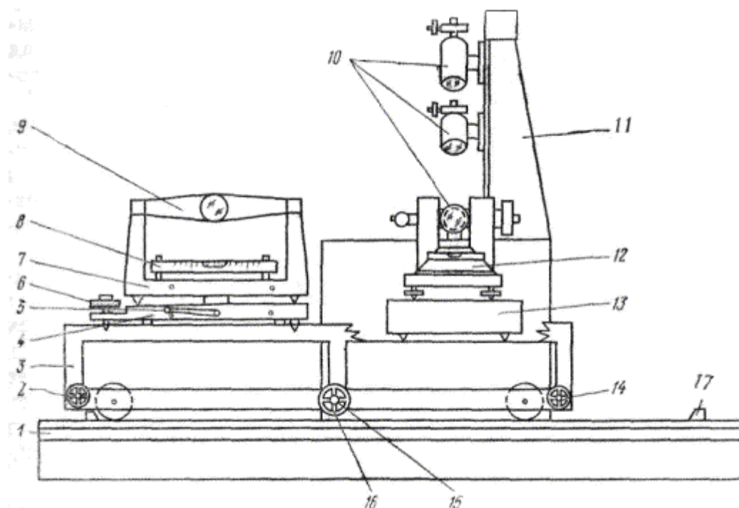
Рис. 10.48. Схема азимутального стенда
