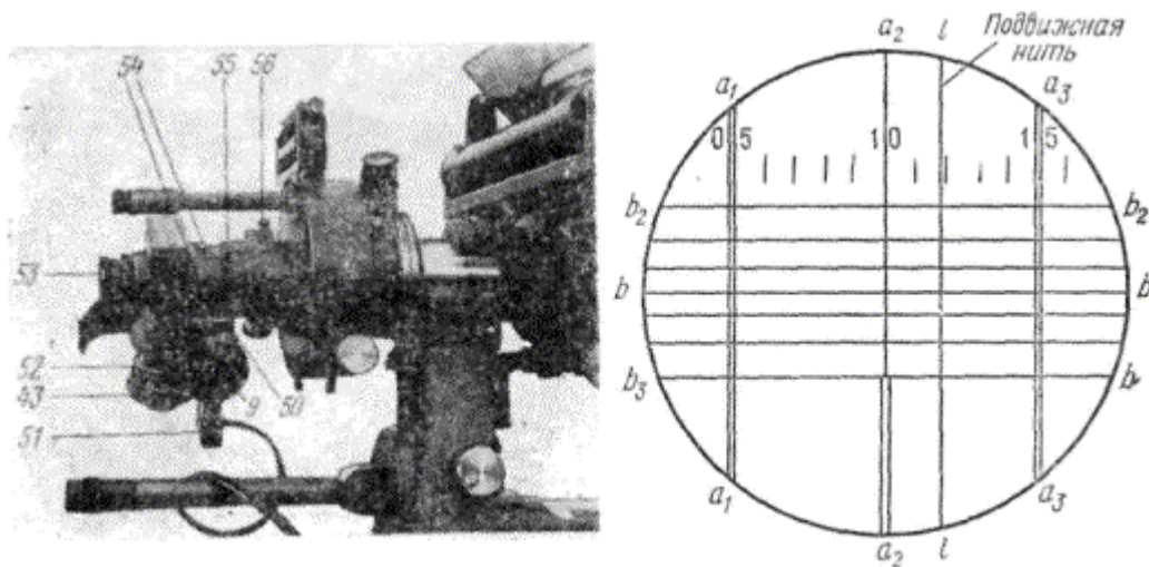
Рис. 10.8. Окулярный конец горизонтальной оси теодолита Т4:
