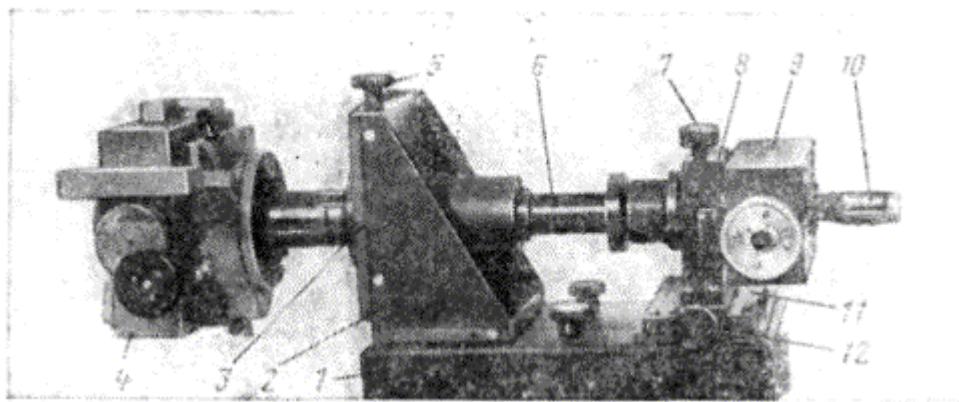
Рис. 10.46. Испытатель микрометрических винтов
