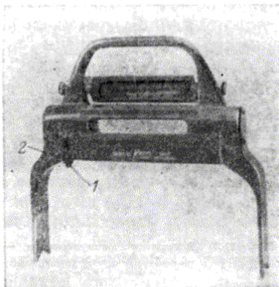
Рис. 11.2. Накладной уровень теодолита ДКМЗ-А
