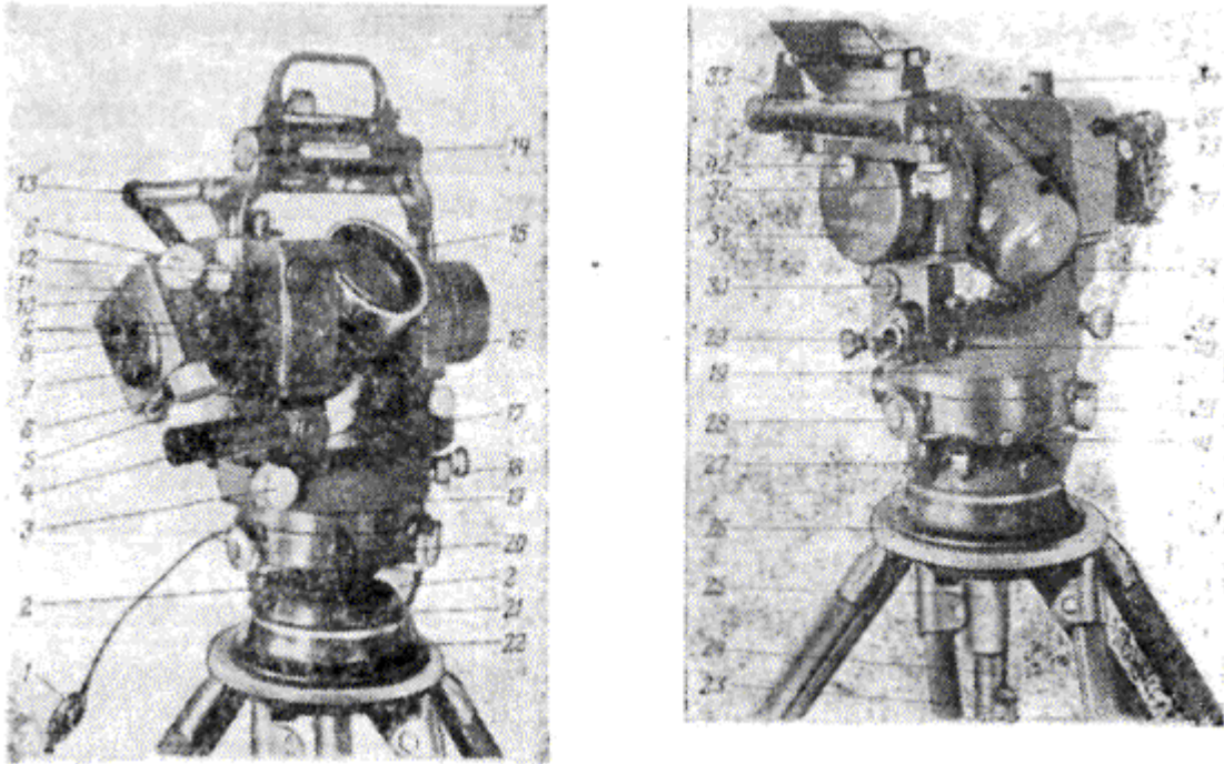
Рис. 10.16. Теодолит ДКМ3-А. Вид со стороны контактного микрометра:
