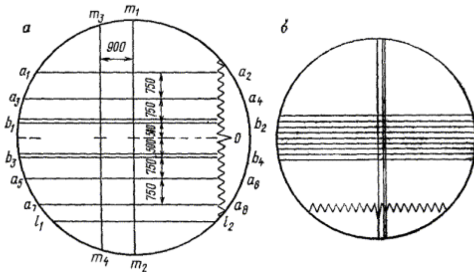
Рис. 10.4. Сетки нитей АУ 2/10:
