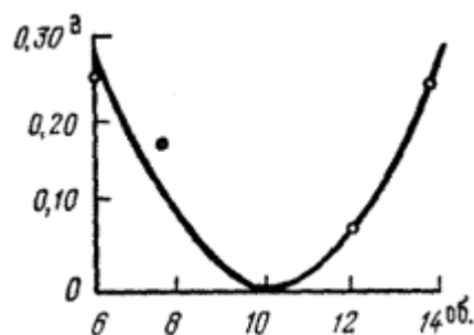
Рис. 11.7. График поправок за ходовые погрешности винта микрометра
