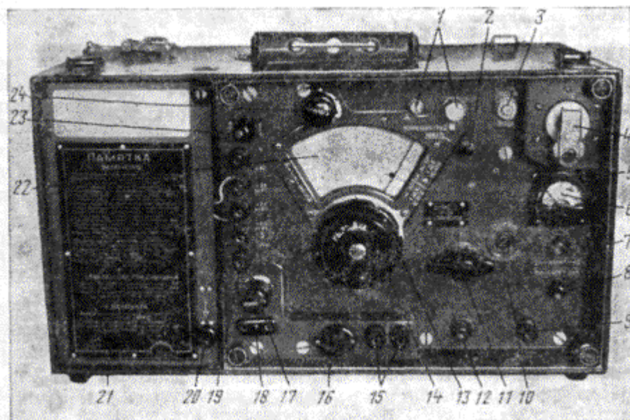
Рис. 10.35. Радиоприемник Р-311
