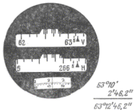
Рис. 10.20. Поле зрения оптического микрометра с отсчетами по вертикальному (сверху), горизонтальному (в середине) кругам и шкалы (внизу) оптического микрометра
