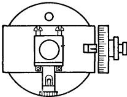
Рис. 10.49. Микрометр с автоколлимационным окуляром
