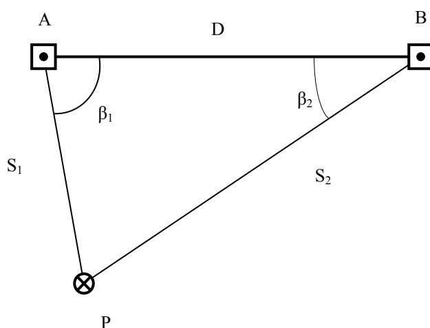
Рис. П.4.1.1 Схема снесения координат пункта наземной сети на рабочий центр способом полярной засечки.
