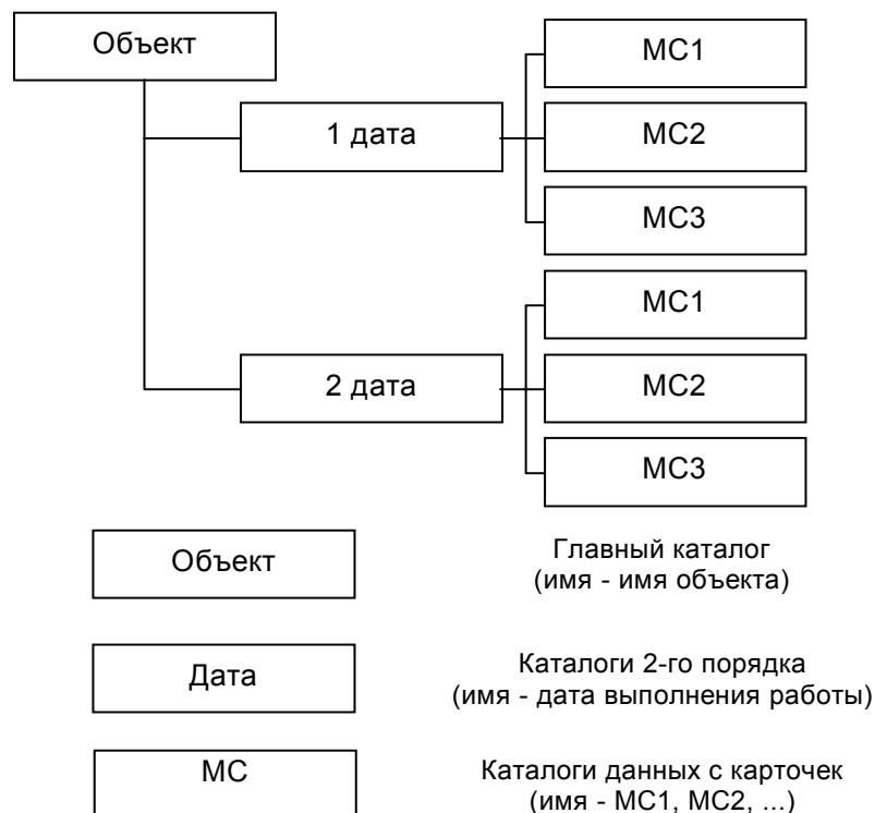
Рис. 5.3.5 Структура каталогов для хранения данных
