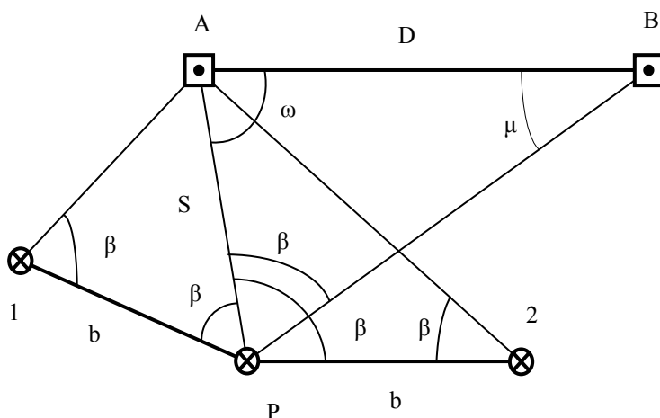
Рис. П.4.1.2 Схема снесения координат пункта наземной сети на рабочий центр способом прямой угловой засечки.
