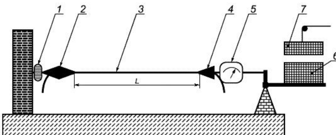
Рисунок 2 - Принципиальная схема установки
