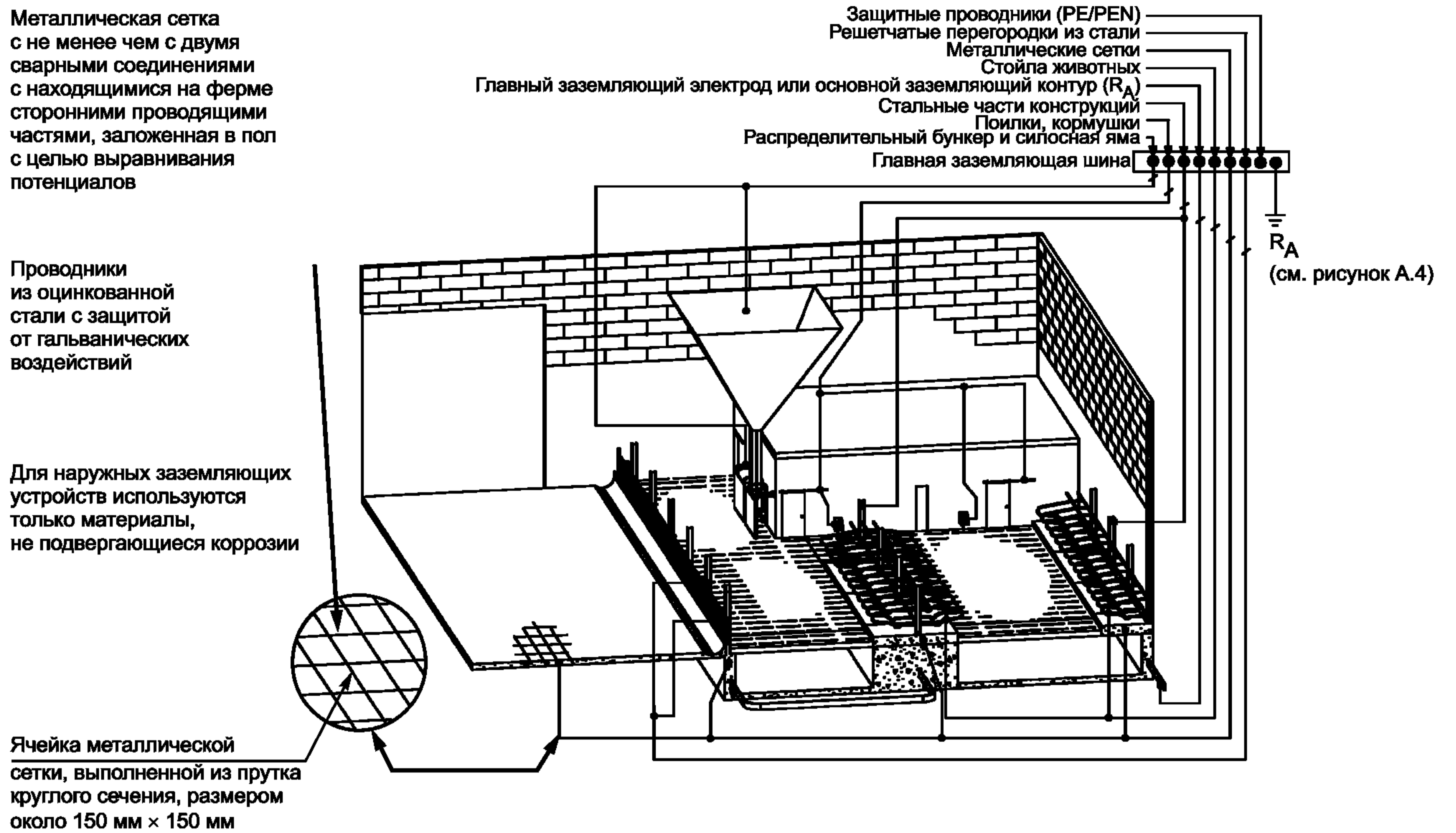
Рисунок А1 — Пример уравнивания потенциалов в коровнике
